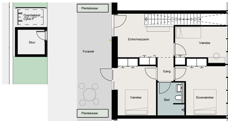
Stueetage
