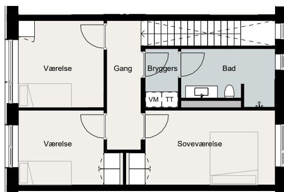
1. sal
